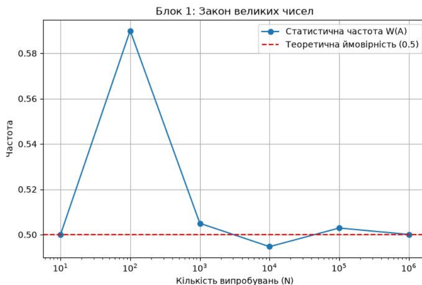
Рис. 2. Графік залежності відносної частоти від кількості випробувань N
